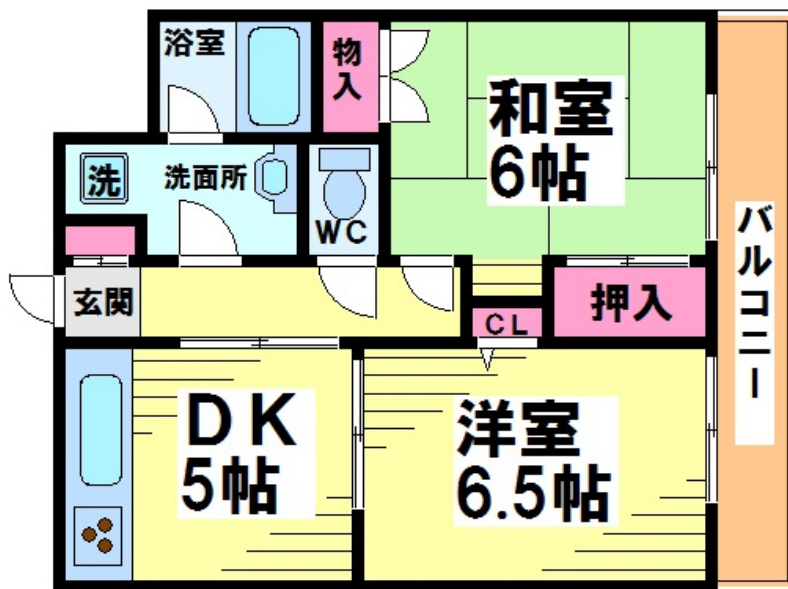
【問取り図】
